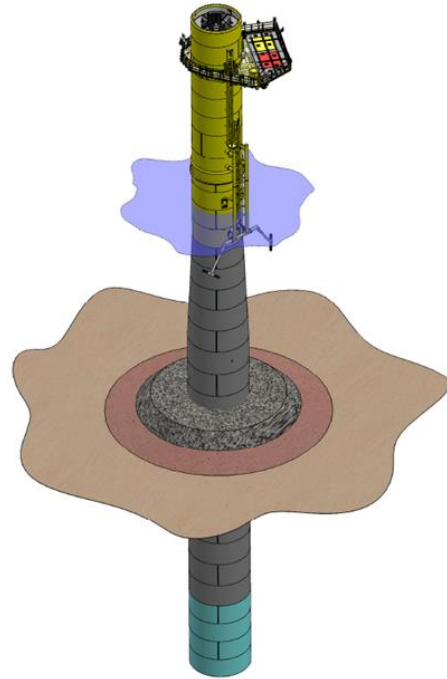
圖 3 基礎採單樁式示意圖
